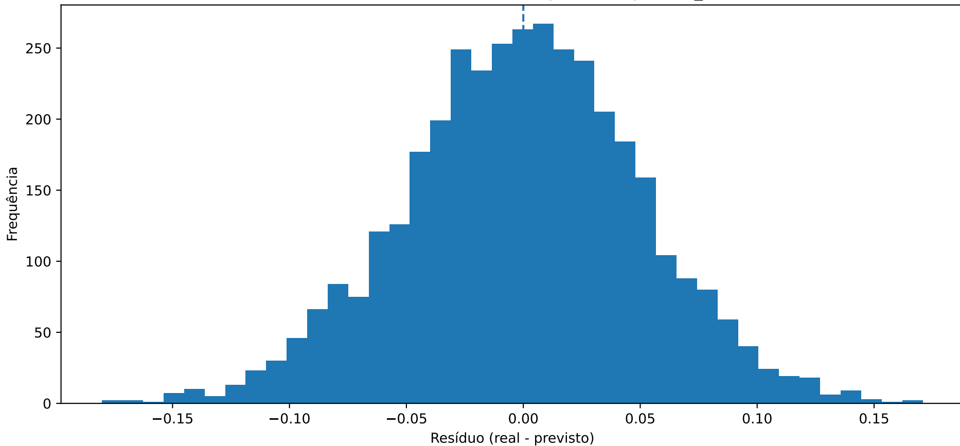
Distribuição dos resíduos — voltagem — Regressao_Linear
